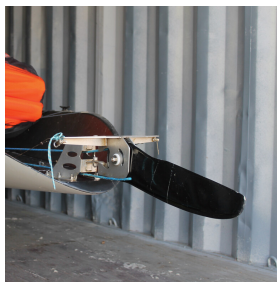
FIGUUR 5.2 Roer in horizontale positie
