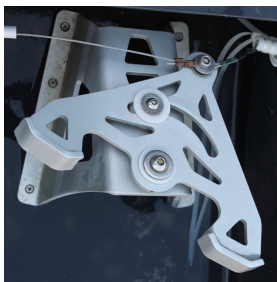
FIGUUR 5.1 Het stuurpedaal van de Barolo
