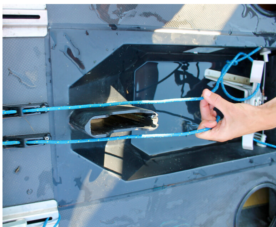
FIGUUR 5.4 Twee lijnen voor de bepaling van de stand van het roer
